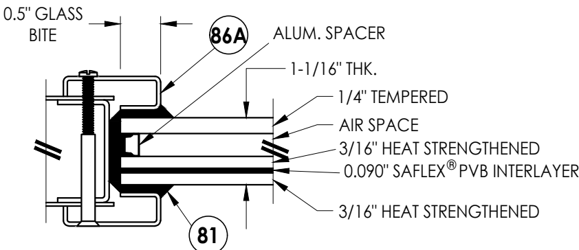
G2 GLAZING DETAIL
